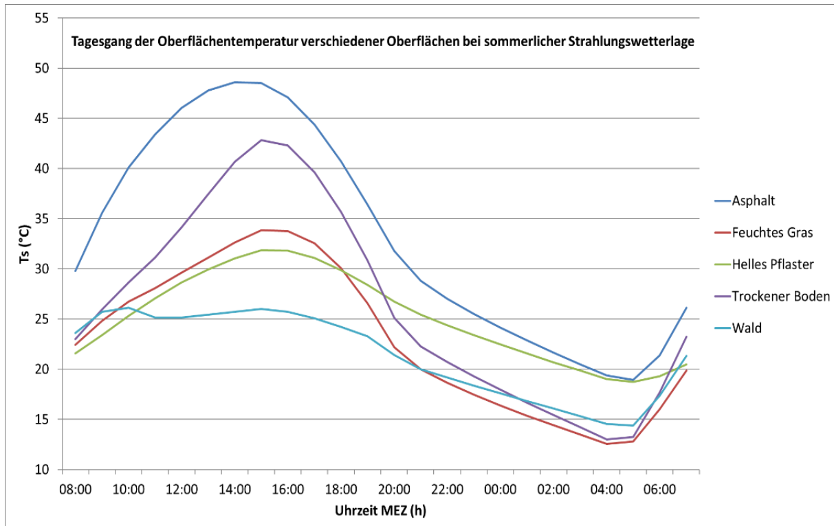
Abb. 4.24 Tagesgang der Oberflächentemperaturen verschiedener Oberflächenmaterialien
