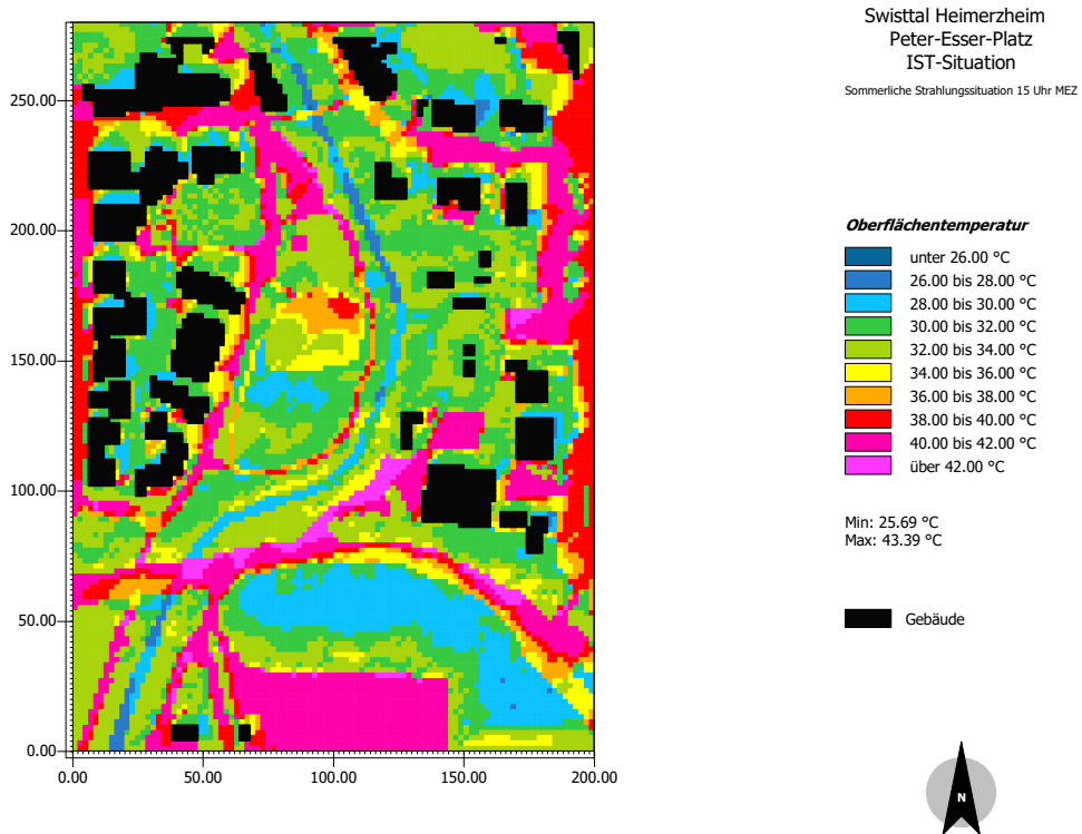
Abb. 4.32 Ergebnis der Berechnungen für die mikroklimatische Situation im IST-Zustand: Oberflächentemperaturen um 15 Uhr
