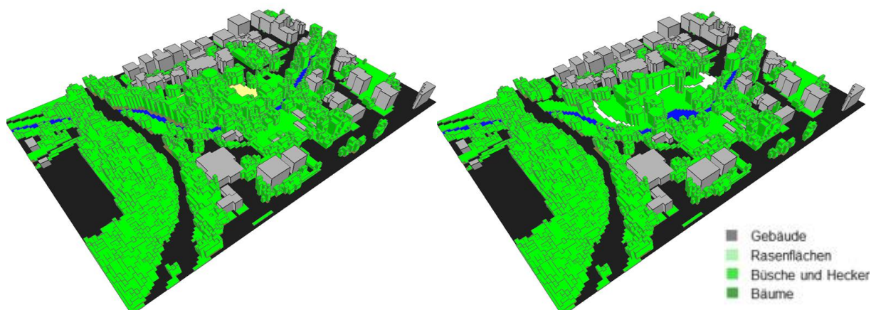
Abb. 4.27 Envi-met Modell für die Berechnung des IST-Zustandes (links) und des Szenarios (rechts) im Untersuchungsgebiet Peter-Esser-Platz
